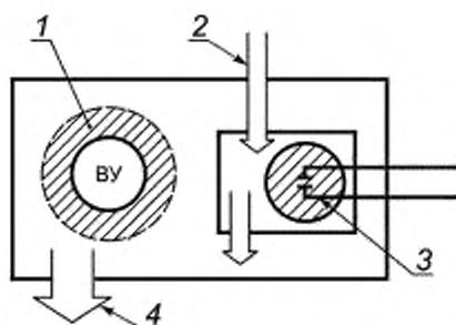
1 — зона, в которой проводится испытание на разбавление; 2 — вход продувочного инертного газа; 3 — потенциальный источник утечки с номинальной зоной разбавления; 4 — выход продувочного газа
