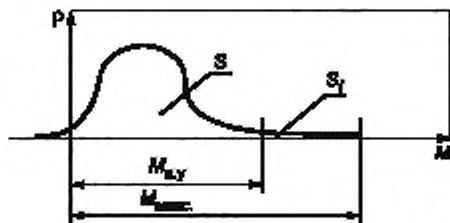
Рисунок 1 — Кривая распределения крутящего момента на ступице колеса
