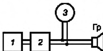
1 — генератор звуковой; 2 — усилитель мощности; 3 — вольтметр (5.10); Гр — громкоговоритель
