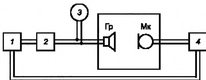
1 — установка для автоматической записи частотной характеристики; 2 — усилитель мощности; 3 — вольтметр (п. 5.4.1); 4 — усилитель микрофонный; Мк — измерительный микрофон; Гр — громкоговоритель.
