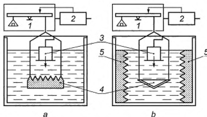
Рисунок F.5 — Компонка Е с поглощающей (а) и вогнутой отражающей (b) мишенями:
