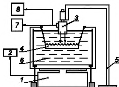
Рисунок F.3 — Компонка В с поглощающей мишенью:
