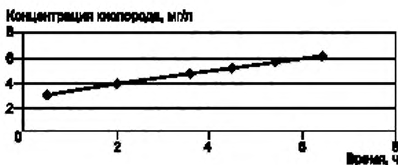
Рисунок D.1 — Изменение во времени концентрации кислорода, растворенного в 200 мл дегазированной методом вакуумирования воды с площадью поверхности 34 \text{ см}^2
