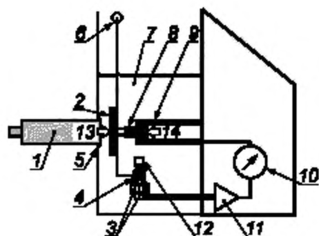
Рисунок F.7 — Компонетка F с поглощающей мишенью:
