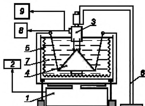
Рисунок F.2 — Компонка В с выгнутой отражающей мишенью:
