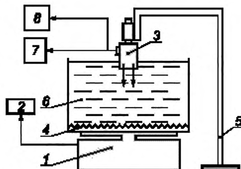
Рисунок F.4 — Компонка С с поглощающей мишенью:
