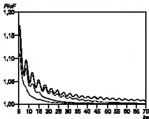
Рисунок Е.2 — Зависимость P/cF от ka для четырех различных псевдотрапециевидных амплитудных распределений: для \epsilon = 0 (поршень) (сплошная кривая), \epsilon = 0,1 (штриховая), \epsilon = 0,25 (точечная), \epsilon = 0,6 (штрихпунктирная)
