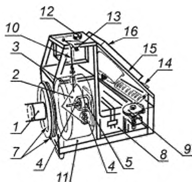
Рисунок F.6 — Компонетка F с выпуклой отражающей мишенью:
