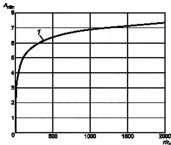
1 — M = 1,3 ; r_0 = 1 м; k = 0,8/340 м -1 ; A_{\text{нлн}} — нелинейное затухание, дБА; r — расстояние от точки источника до точки наблюдения, м
