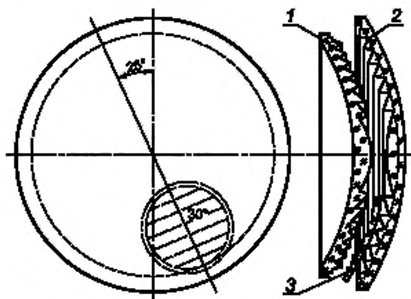
1 — светофильтр-линза СЛ 139; 2 — линза ЛС 160; 3 — отклоняющая вставка OB 52
