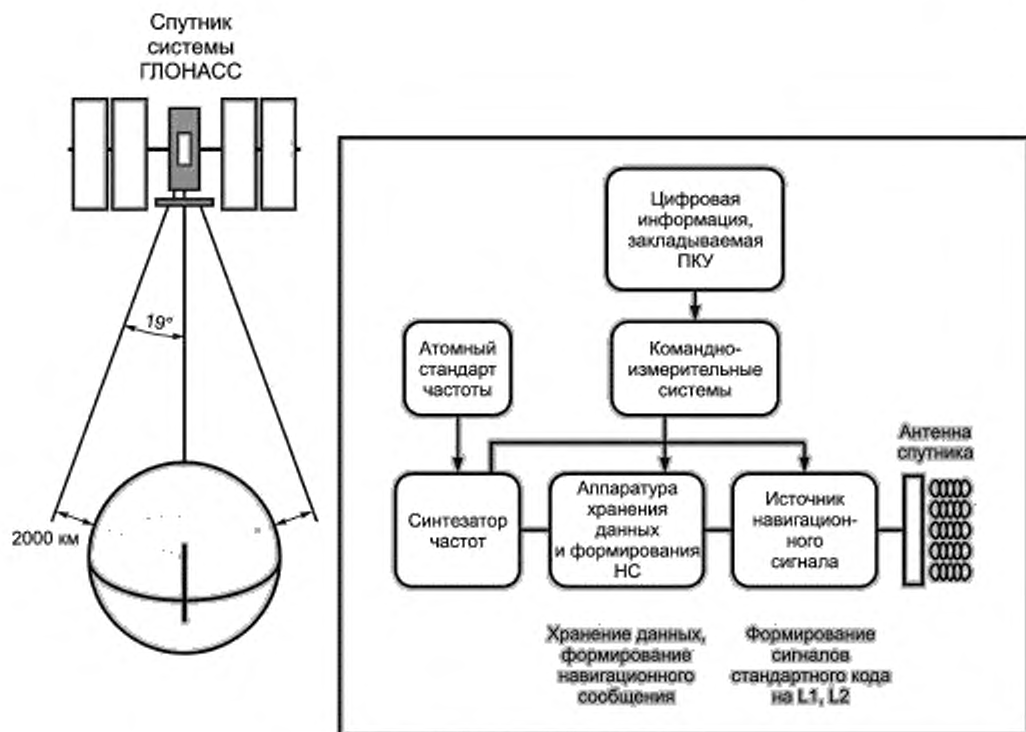
Рисунок А.1 — Процесс генерации сигналов на спутнике
