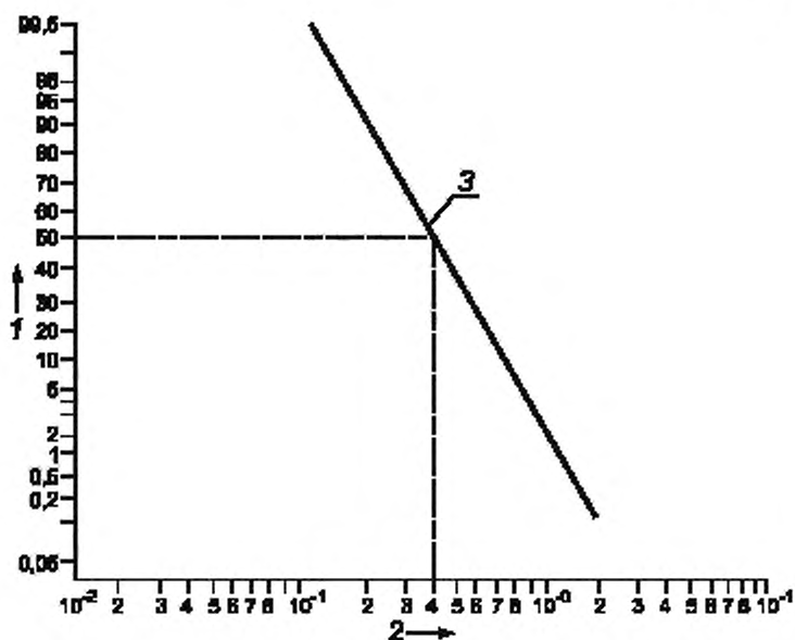
Рисунок 6 — Распределение частиц аэрозоля парафинового масла по размерам
