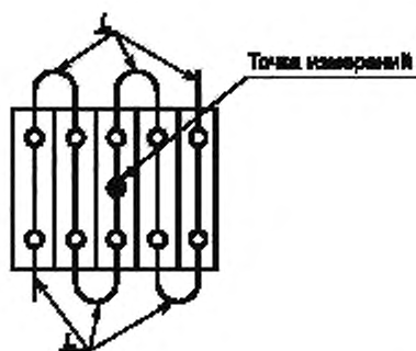
Рисунок 3 — Схема для испытания на превышение температуры (группа а)
