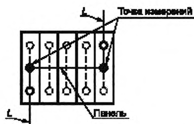
Рисунок 4 — Схема для испытания на превышение температуры (группа б)
