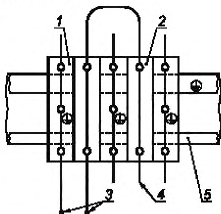
1 — клеммная колодка защитных проводников; 2 — клеммная колодка по ГОСТ Р 50030.7.1; 3 — испытательное напряжение; 4 — концы проводников; 5 — металлическое основание
