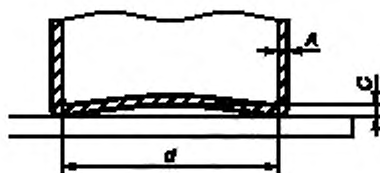
A — толщина дна и стенок сосуда ( 2 \pm 0,5 ) мм; C — максимальная вогнутость, d — диаметр плоской поверхности дна
