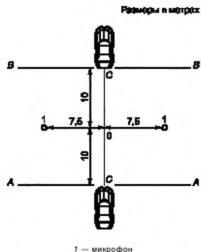
Рисунок 2 — Местоположения микрофонов
