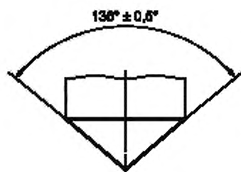
Рисунок 1 — Угол алмазной пирамиды
