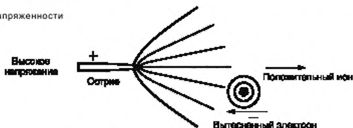
Рисунок 10 — Коронная ионизация — положительная
