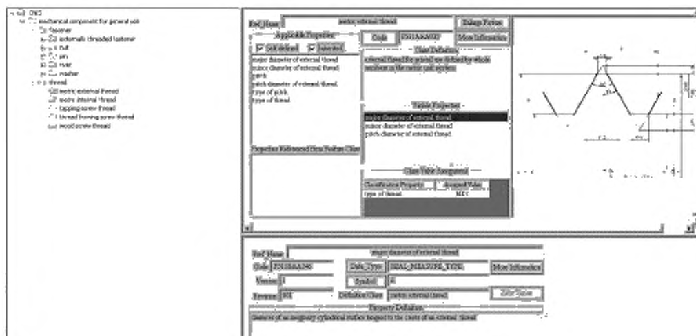
Рисунок 4 — Характеристический класс резьб по ISO 13584-511
