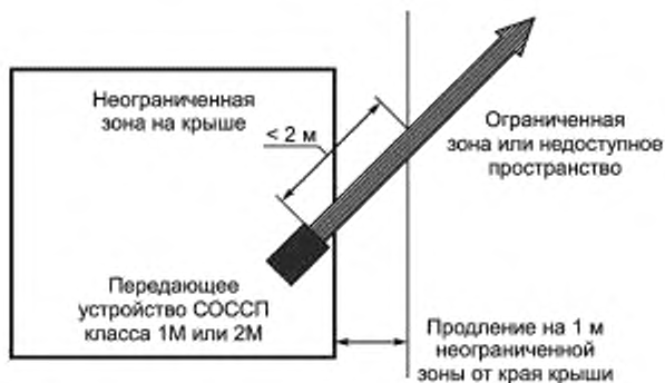
Рисунок 4 — Передающее устройство лазеров класса 1М или 2М вблизи края крыши в неограниченной зоне
