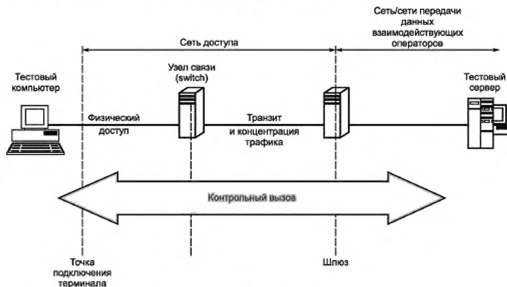
Рисунок Б.1 — Измерительная установка
