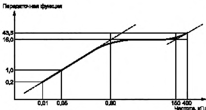
Рисунок 1 — Передаточная функция
