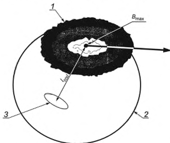
Рисунок D.1 — Измерение магнитной индукции
