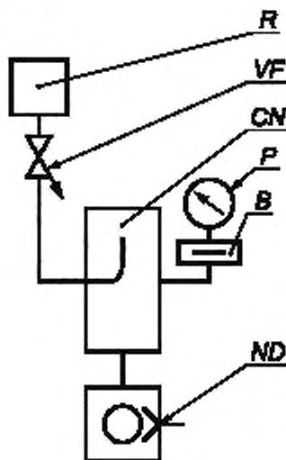
R — устройство для измерения потока, VF — клапан-напекатель; CN — измерительная камера, P — вакуумметр; B — охлаждаемая ловушка; ND — испытываемый насос
