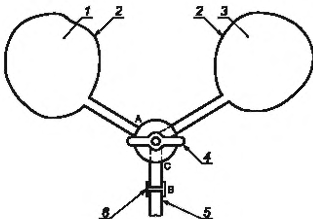
1 — ПГС; 2 — газовые емкости; 3 — чистый воздух; 4 — двухходовой кран; 5 — пробитый зонд или газовый вход прибора; 6 — устройство для подключения прибора
