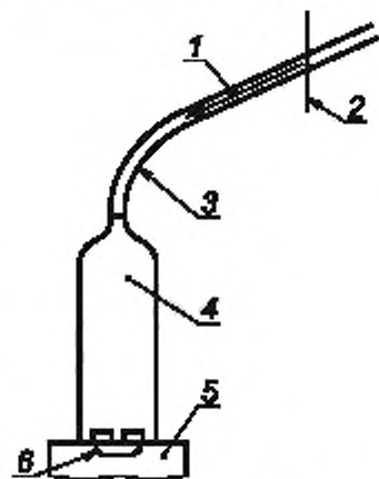
1 — чистый воздух или ПГС; 2 — расхономер; 3 — гибкая трубка; 4 — трубчатый аппликатор; 5 — газоанализатор (датчик); 6 — вход газоанализатора (датчика)
