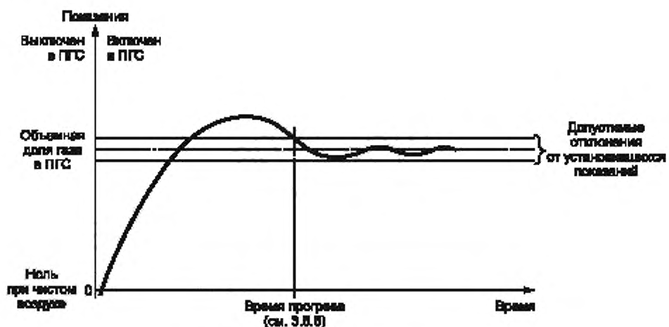
Рисунок 2 — Время прогрева в ПГС
