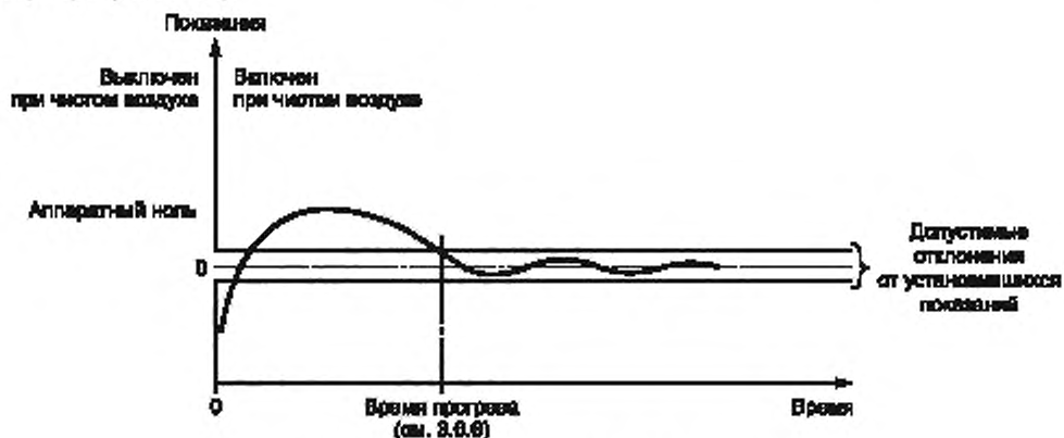
Рисунок 1 — Время прогрева в чистом воздухе
