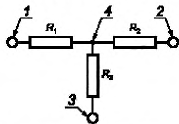
1, 2, 3 и 4 — клеммы для подключения меры; R_1 , R_2 и R_3 — меры активного электрического сопротивления
