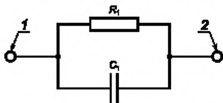
1 и 2 — клеммы для подключения меры; R_1 — мера активного электрического сопротивления; C_1 — мера электрической емкости
