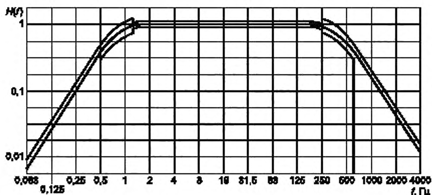
Рисунок 2 — Амплитудно-частотная характеристика измерительной цепи
