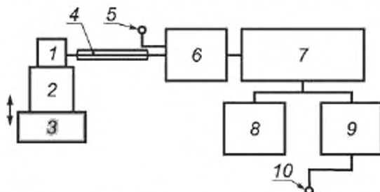
1 -- датчик вибрации; 2 -- система крепления; 3 -- вибрирующая поверхность; 4 -- соединительный кабель; 5 -- электрический вход; 6 -- устройство согласования входного сигнала; 7 -- фильтр; 8 -- показывающее устройство с устройством выделения и хранения пикового значения; 9 -- устройство согласования выходного сигнала; 10 -- аналоговый/цифровой выход
