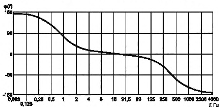
Рисунок 3 — Фазочастотная характеристика измерительной цепи
