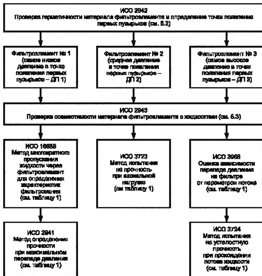
Рисунок 1. Последовательность испытаний
