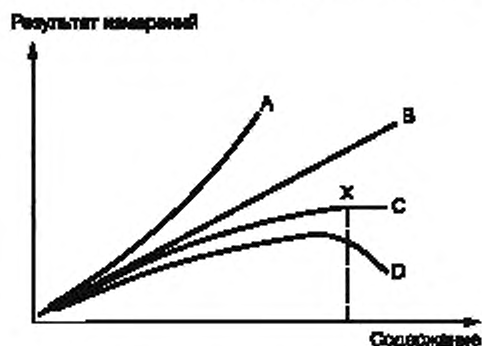
Рисунок 1 — Зависимость результата измерения от содержания загрязняющего вещества
