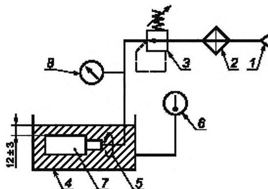
1 — устройство подачи сжатого воздуха; 2 — фильтр для сжатого воздуха; 3 — регулятор давления; 4 — ванна для испытаний; 5 — испытательная жидкость; 6 — прибор для измерения температуры; 7 — испытываемый фильтроэлемент; 8 — прибор для измерения давления
