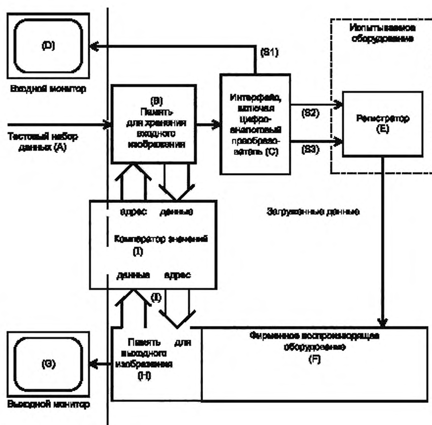
Рисунок 1 — Блок-схема испытаний
