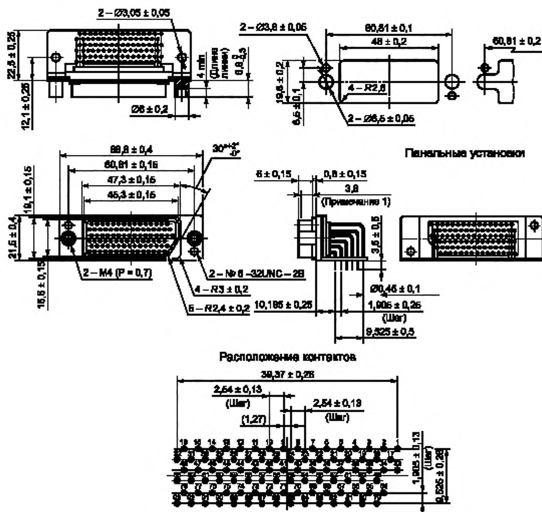
Рисунок 11 — 93-й контактный разъем (розетка)
