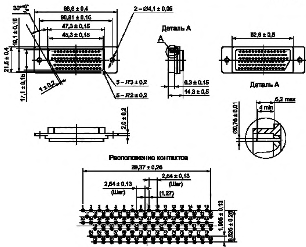
Рисунок 10 — 93-й контактный разъем (вилка)
