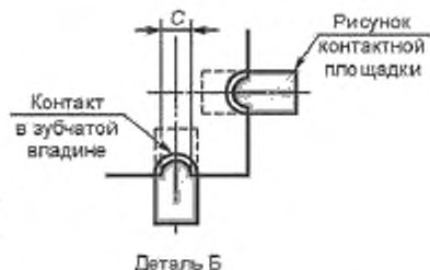
Рисунок 33 — Установка кристаллоносителя: заданное состояние
