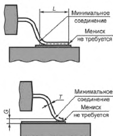
Рисунок А.4 — Совмещение допустимое состояние
