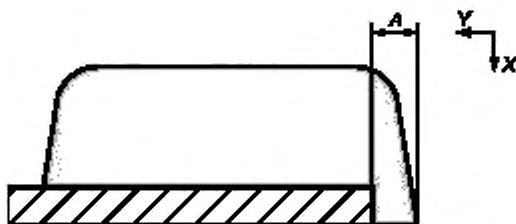
Рисунок 2 — Контур и сечение паяльной пасты: допустимое состояние
