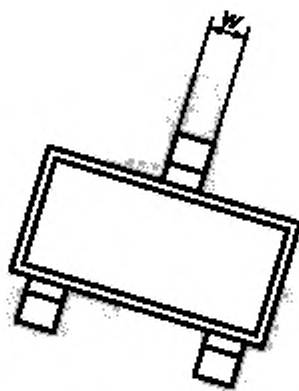
Рисунок 11 — Установка дискретного компонента: недопустимое состояние
