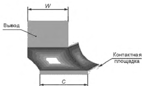
Рисунок А.29 — Галтель припоя: заданное состояние
