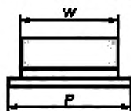
Рисунок 30 — Установка компонента с контактами на нижней поверхности: заданное состояние
