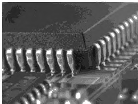
Рисунок А.11 — Галтель припоя: допустимое состояние
