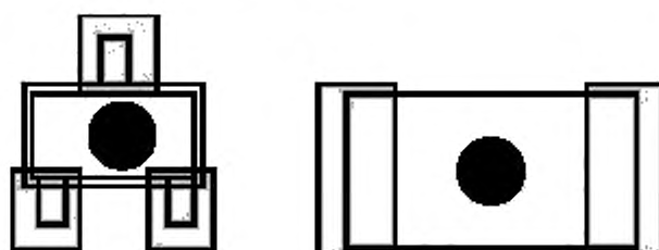
Рисунок 6 — Контур и качество нанесения клея: заданное состояние
