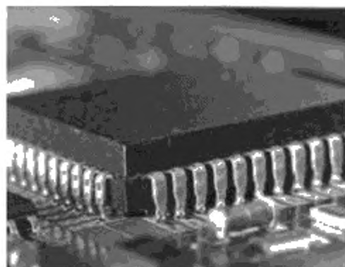
Рисунок А.9 — Галтель припоя: заданное состояние
