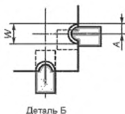
Рисунок 34 — Установка кристаллоносителя: допустимое состояние
