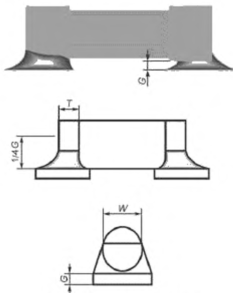
Рисунок А.19 — Галтель припоя: допустимое состояние
