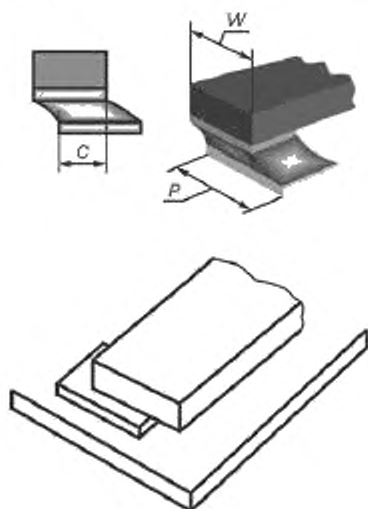
Рисунок А.23 — Галтель припоя: допустимое состояние
