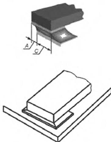
Рисунок А.24 — Совмещение: допустимое состояние
