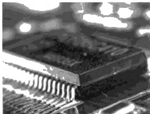
Рисунок А.1 — Галтель припоя: заданное состояние
