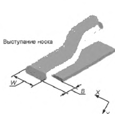
Рисунок 19 — Смещение круглых и расплюснутых выводов на контактной площадке: допустимое состояние
