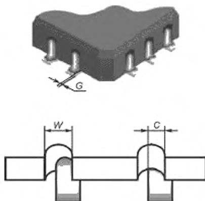
Рисунок А.27 — Галтель припоя: допустимое состояние
