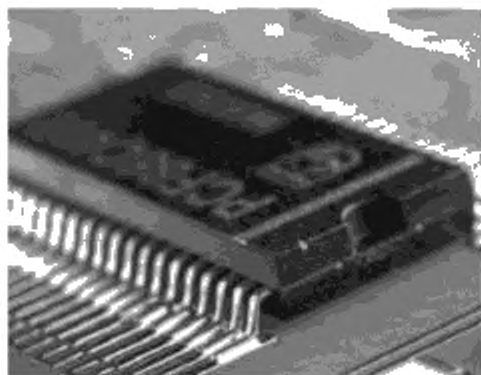
Рисунок А.3 — Галтель припоя: допустимое состояние
