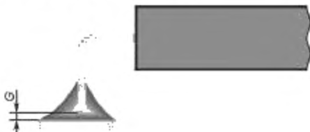
Рисунок А.32 — Совмещение: допустимое состояние
