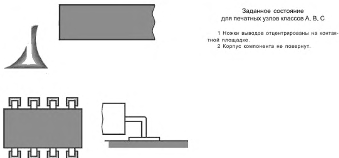
Рисунок 36 — Установка компонента с выводами для пайки встык: заданное состояние
