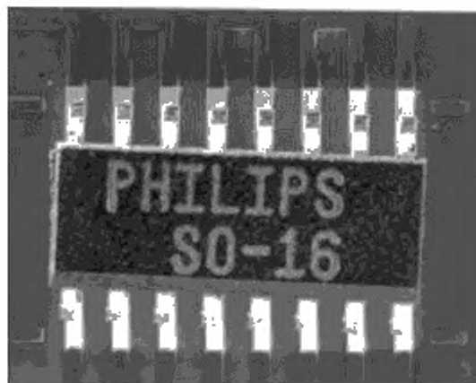
Рисунок 12 — Установка корпусов микросхем с выводами в виде крыла чайки на две стороны: заданное состояние
