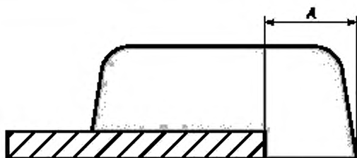
Рисунок 3 — Контур и сечение паяльной пасты: недопустимое состояние
