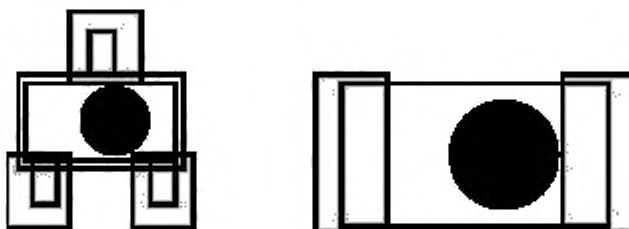
Рисунок 7 — Нанесение клея: допустимое состояние
