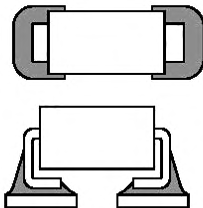
Рисунок А.34 — Смещение: заданное состояние
