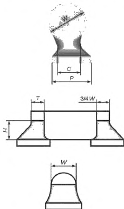
Рисунок А.17 — Галтель припоя: заданное состояние
