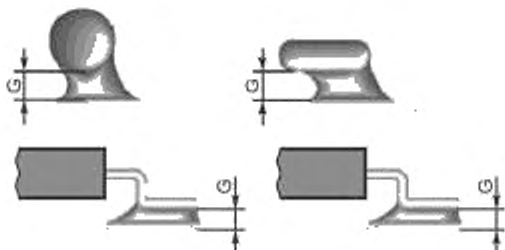
Рисунок А.8 — Совмещение: допустимое состояние
