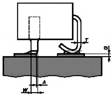
Рисунок А.12 — Совмещение: допустимое состояние
