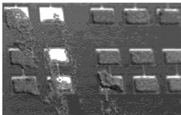
Рисунок 5 — Смазанная паста: недопустимое состояние
