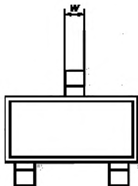
Рисунок 10 — Установка дискретного компонента: допустимое состояние
