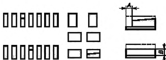
Рисунок 3 — Контур и сечение паяльной пасты: недопустимое состояние
