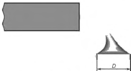
Рисунок А.31 — Галтель припоя: допустимое состояние
