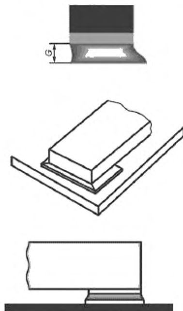
Рисунок А.21 — Галтель припоя: заданное состояние
