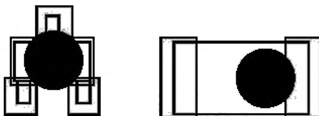
Рисунок 8 — Нанесение клея: недопустимое состояние
