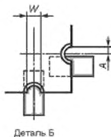
Рисунок 35 — Установка кристаллоносителя: недопустимое состояние
