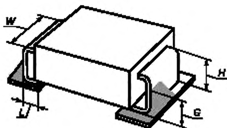
Рисунок А.35 — Галтель припоя: допустимое состояние
