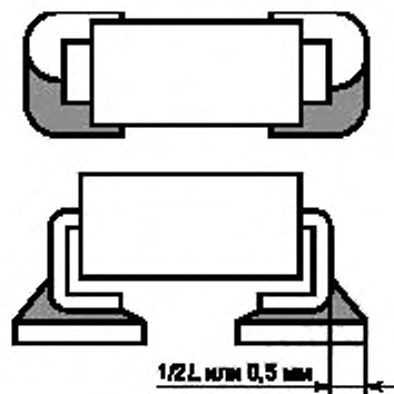
Рисунок А.36 — Совмещение: допустимое состояние
