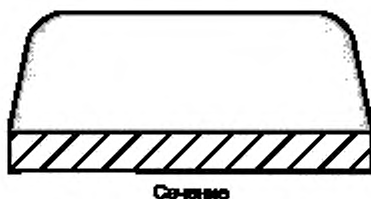
Рисунок 1 — Контур и сечение паяльной пасты: заданное состояние
