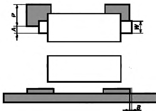
Рисунок 41 — Установка компонента с ленточными L-образными выводами, отформованными под корпус: недопустимое состояние
