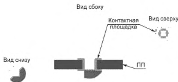
Рисунок 19 — Галтели припоя: допустимое состояние
