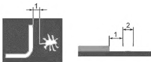
Рисунок 59 — Шарик или бусинки припоя: недопустимое состояние
