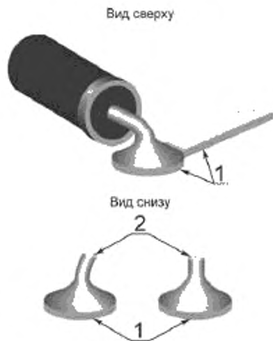
Рисунок 72 — Обнажение основного металла: допустимое состояние
