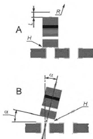
Рисунок 36 — Компоненты с осевыми выводами, вертикальная установка с зазором: недопустимое состояние
