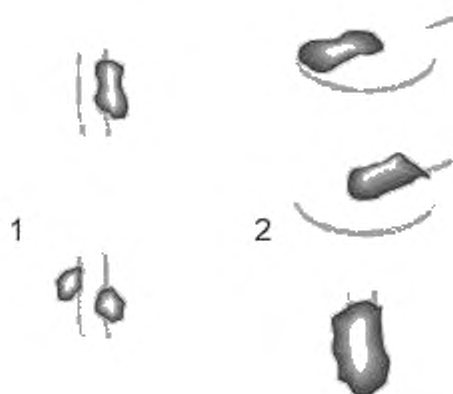
Рисунок 71 — Запаянные выводы, металлизированные сквозные отверстия: допустимое состояние
