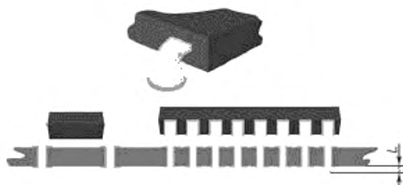
Рисунок 31 — Корпуса DIP: заданное состояние
