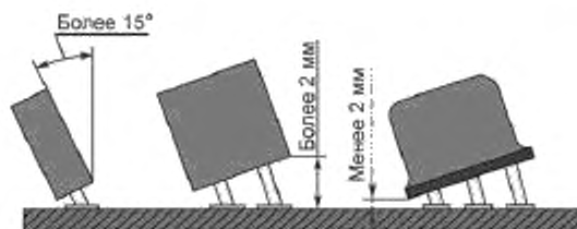
Рисунок 28 — Компоненты с радиальными выводами, вертикальный монтаж: виды состояний
