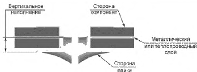
Рисунок 64 — Тепловой слой, наполнение отверстия припоем: виды состояний
