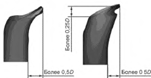
Рисунок 10 — Обрезка вывода: недопустимое состояние
