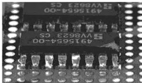
Рисунок 53 — DIP-корпус: допустимое состояние
