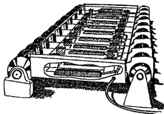
Рисунок А.5 — Комплексное испытательное устройство с вращающимися натяжными барабанами
