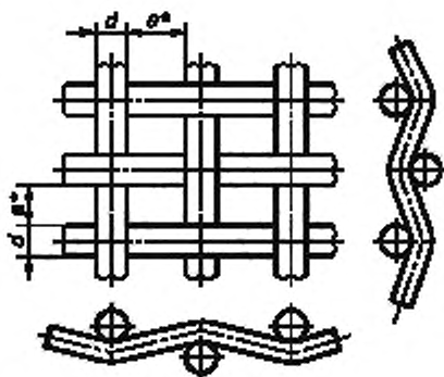
Рисунок 1 — Сетка типа СПП
