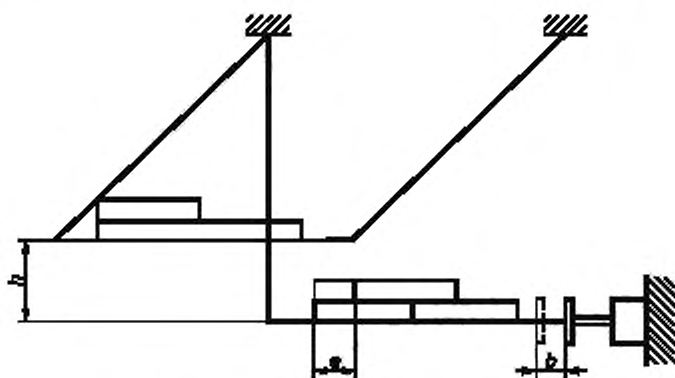
Рисунок 2 — Метод испытания маятниковым прибором
