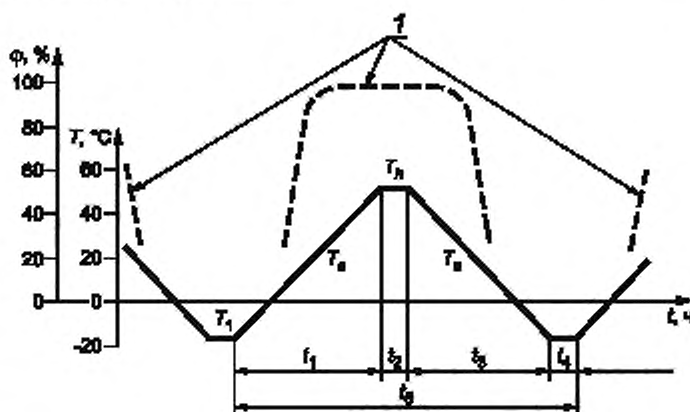
\varphi — относительная влажность в течение температурного цикла; T_n — температура выдержки, равная (53,0 \pm 1,0) °C; T_l — температура выдержки, равная минус (18,0 \pm 2,0) °C; T_g — перепад температур, равный (14 \pm 2,0) °C в течение часа; t_1 - t_5 — интервалы времени; \varphi — влажность
