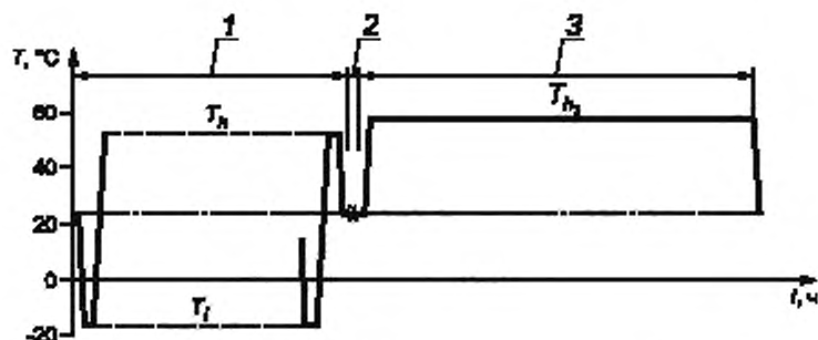
1 — первый этап испытаний; 2 — второй этап испытаний; 3 — третий этап испытаний; T_n — температура выдержки, равная (53,0 \pm 1,0) °C; T_{n2} — температура выдержки, равная (58,0 \pm 0,5) °C; T_l — температура выдержки, равная минус (18,0 \pm 2,0) °C
