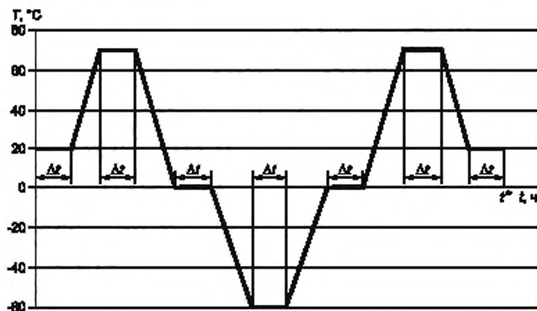
Рисунок 1 — График испытаний одного цикла
