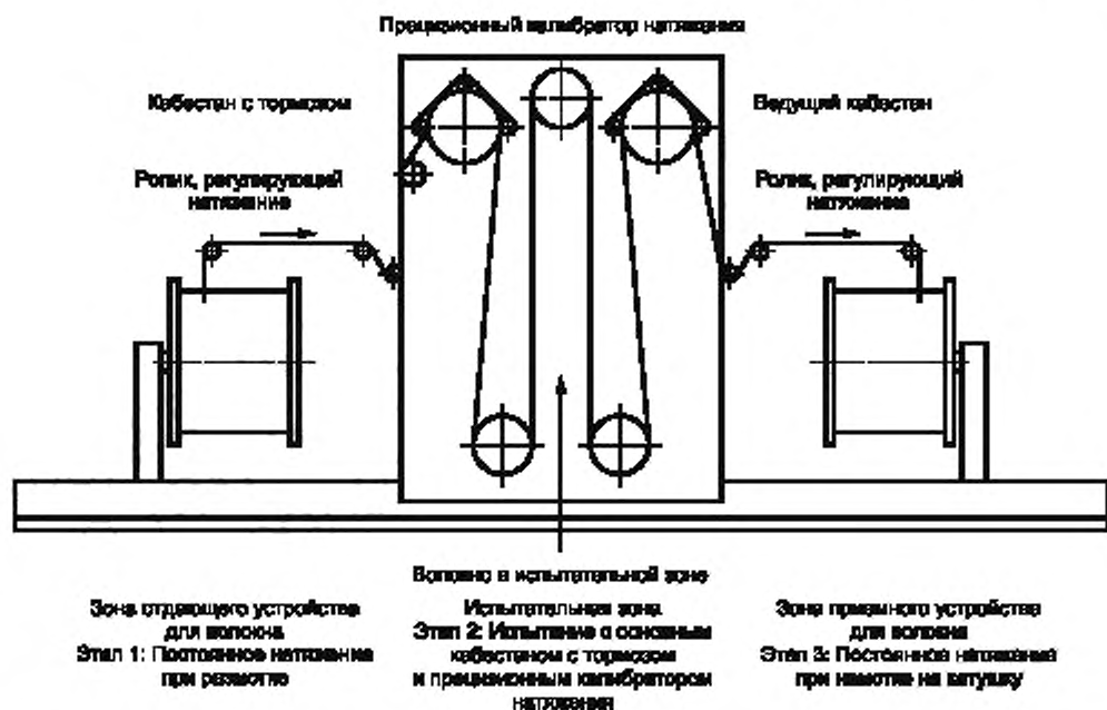
Рисунок 1 — Испытательное устройство с кабестаном, снабженным тормозом
