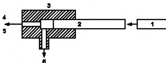
1 — атмосфера испытаний по ГОСТ ИСО 3402; 2 — сменный калибр; 3 — соединительный патрубкок; 4 — объемный поток воздуха; 5 — источник всасывания ( 17,5 \pm 0,3 см 3 /с); 6 — место присоединения преобразователя давления
