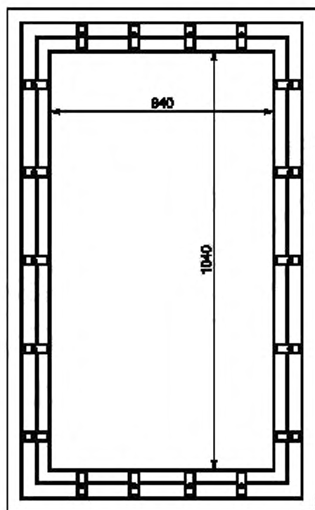
Рисунок В.2 — Наружная рама
