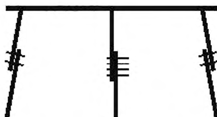
Рисунок 2 — Схема трапециевидной крепи с одной дополнительной центральной стойкой (боковые стойки могут быть криволинейными)
