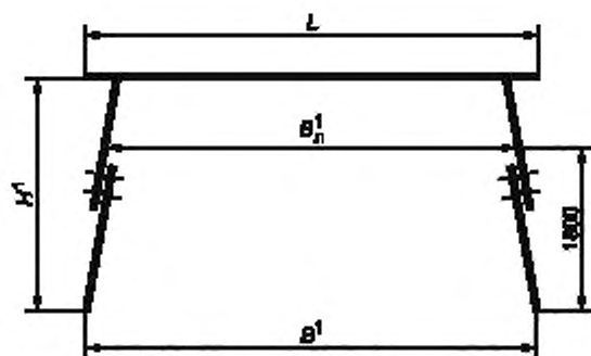
Рисунок 1 — Схема трапециевидной крепи (стойки могут быть криволинейными)
