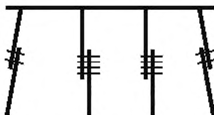
Рисунок 3 — Схема трапециевидной крепи с двумя дополнительными центральными стойками (боковые стойки могут быть криволинейными)
