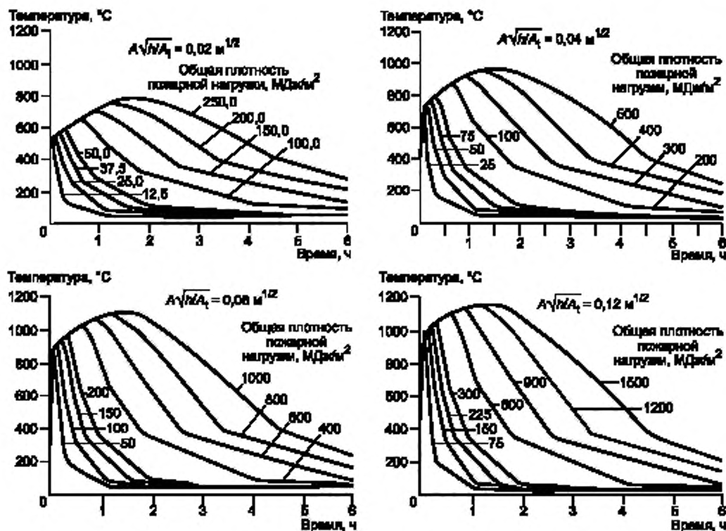
Рисунок 9 — Примеры зависимости средневolumной температуры газа от времени при объемном пожаре в помещении при различных значениях плотности пожарной нагрузки и коэффициента проемности [10]
