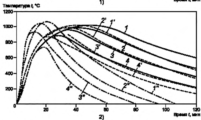
Рисунок 9е — Результаты расчета изменения параметров при пожаре в помещении объемом V = 50,3 \text{ м}^3 для температур поверхности перекрытия (9е-1) и среднеобъемной (9е-2) ([5])
