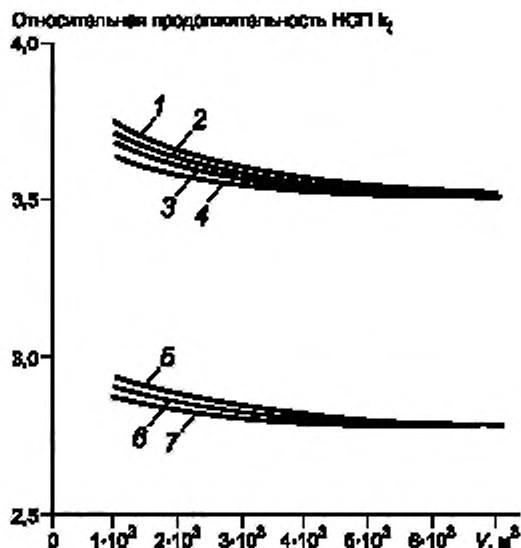
Рисунок бв — Зависимость относительной продолжительности начальной стадии пожара (НСП) от объема V и высоты H помещения [29]
