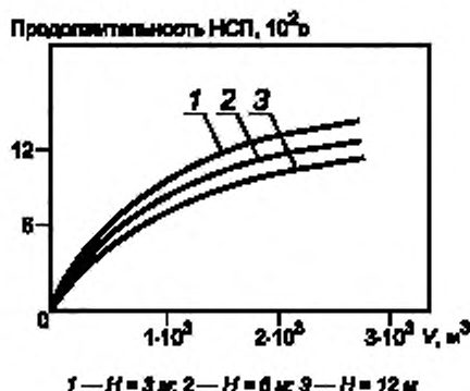
Рисунок бб — Зависимость минимальной продолжительности начальной стадии пожара (НСП) от объема V и высоты H помещения
