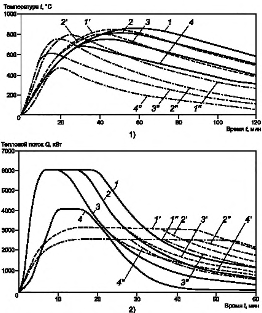
Рисунок 9а — Результаты расчета изменения параметров при пожаре в помещении объемом V = 50,3 \text{ м}^3 для температуры поверхности стены (9а-1) и теплового потока (9а-2) [5]
