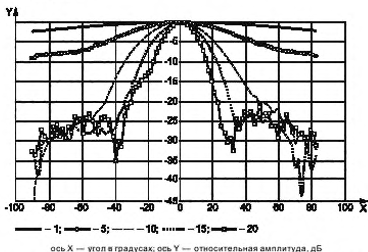
Рисунок А.2 — Характеристики направленности 0,2 мм — зондового гидрофона
