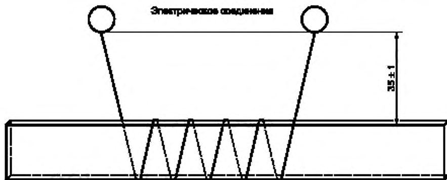
Рисунок 2 — Пример намотки проволоки на испытуемый образец
