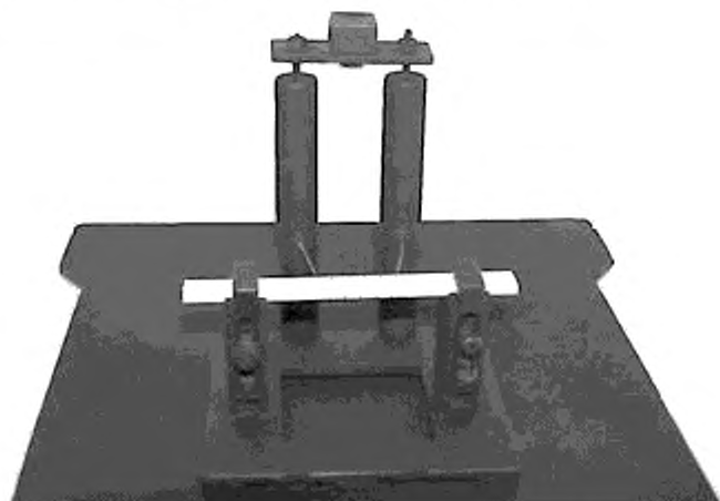
Рисунок 1 — Пример монтажа испытательного зажимного приспособления
