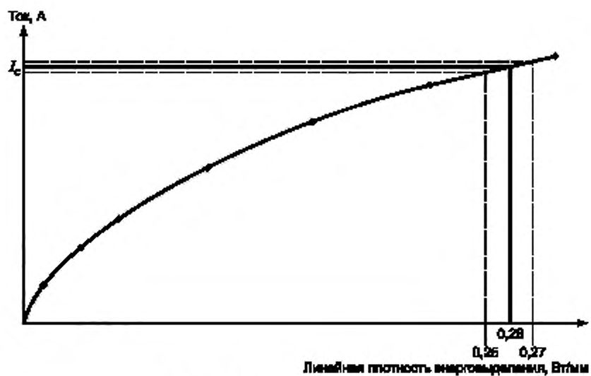
Рисунок А.2 — Калибровочная кривая
