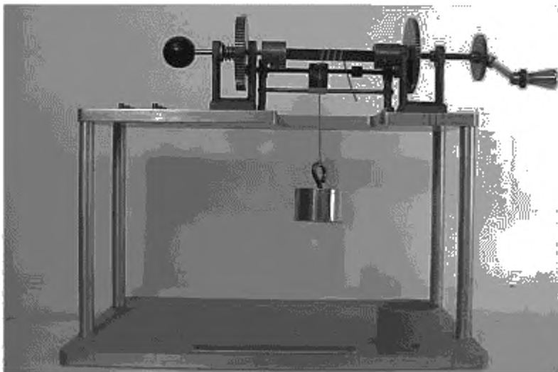
Рисунок 4 — Пример намоточного устройства
