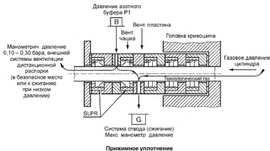
Прижимное уплотнение
