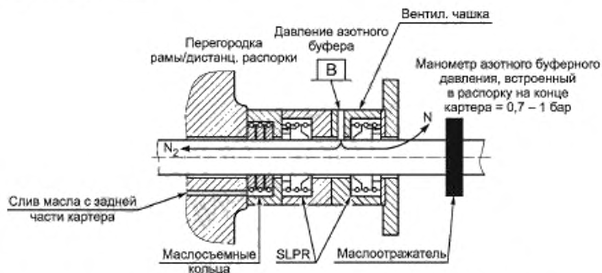
Уплотнение с маслосъемным кольцом (с N 2 буфером)
