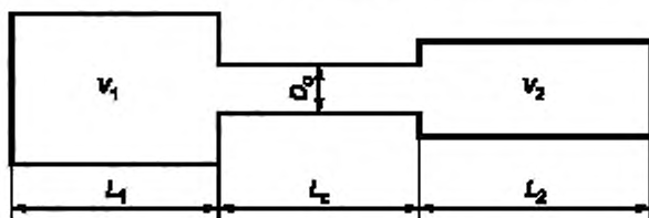
Рисунок О.1 — Несимметричный фильтр
