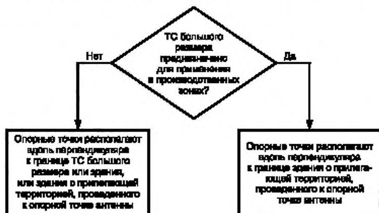
Рисунок 1 — Подход к определению опорных точек при измерениях напряженности поля ИРП от порта корпуса ТС больших размеров в условиях эксплуатации
