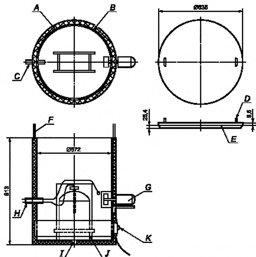
А — изоляция толщиной 25 мм; В — барабан без дна, 220 л; С — труба, 19 мм; D — стержень с петлей, 9,6 мм; E — изоляция на стальном покрытии; F — контрольный кабель, 3 мм; G — вентилятор; H — термодары и контрольные приборы, I — дренаж, J — угловая стойка, 25 мм, K — нагреватель барабана, 2 кВт
