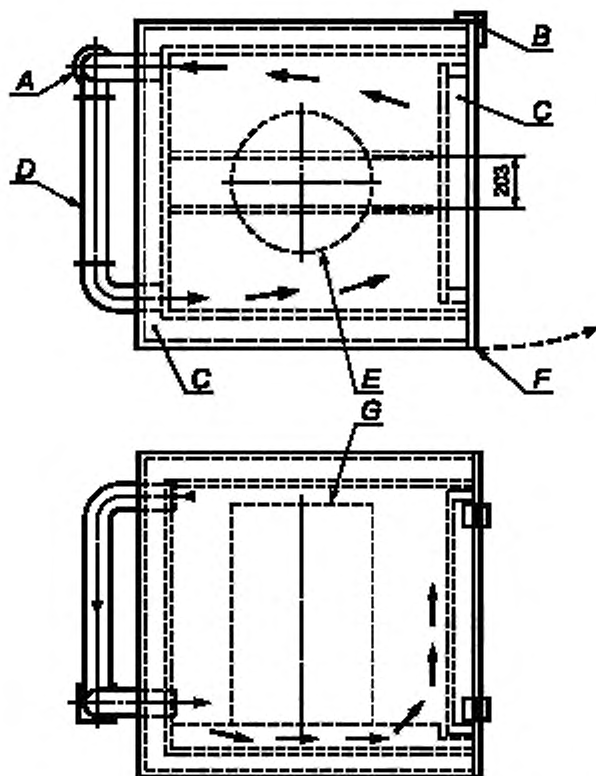
А — вентилятор, В — шарниры; С — изоляция; D — нагреватель; E — барабан; F — зазор; G — барабан (например, 0,58 × 0,89 м)
