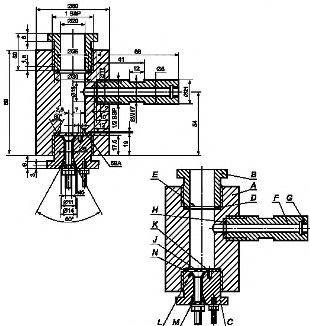
А — корпус сосуда высокого давления; В — фиксирующая пробка разрывной мембраны; С — запальная пробка; D — мягкая свинцовая прокладка; Е — разрывная мембрана; F — боковое ответвление; G — резьба датчика давления; H — медная прокладка; J — изолированный электрод; K — заземленный электрод; L — изоляция; M — стальной конус; N — паз смещения прокладки
