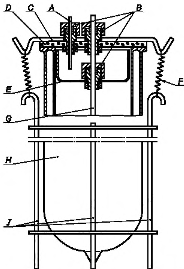
A — капиллярная трубка из ПТФЭ; B — специальные заворачивающиеся заглушки (из ПТФЭ или алюминия) с уплотнительными кольцами; C — металлическая планка; D — стеклянная крышка; E — основание стеклянного резервуара; F — пружина; G — стеклянная защитная трубка; H — сосуд Дьюара; J — стальное поддерживающее устройство
