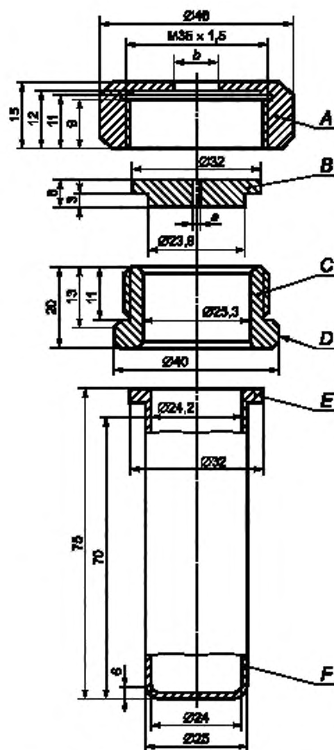
A — гайка ( b = 10,0 или 20,0 мм), рассчитанная на гаечный ключ 41; B — пластина с отверстием ( a = 1,0 \times 20,0 мм в диаметре); C — резьбовое кольцо; D — фаски для гаечного ключа 36; E — фланец; F — трубка
