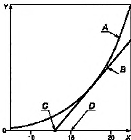
А — кривая тепловыделения; В — прямая с градиентом, равным скорости теплоотдачи, проведенная по касательной к кривой тепловыделения; С — критическая температура окружающей среды (пересечение линии теплоотдачи с абсциссой); D — ТСУР — критическая температура окружающей среды, округленная до более высокого значения, кратного 5 °С; X — температура; Y — тепловой поток на единицу массы
