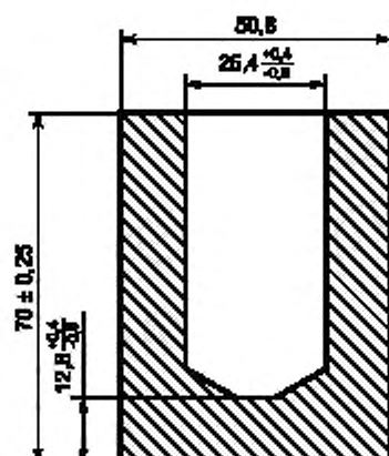
Рисунок 14 — Установка для проведения испытания по модифицированному методу Трауцля
