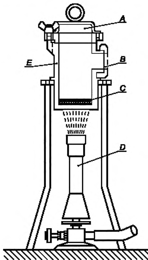
А — разрывная мембрана; В — пластина с отверстием; С — опытный образец; D — горелка типа «Теклю»; E — сосуд высокого давления внутренним диаметром 50 мм и внутренней высотой 94,5 мм
