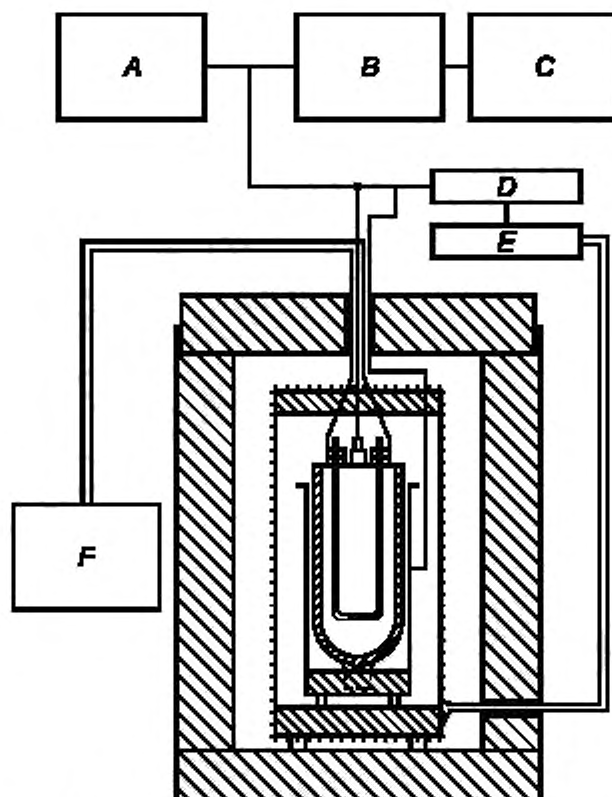
A — многоотсчетный регистратор и регулятор температуры (10 мВ); B — наружная установка на ноль; C — записывающее устройство высокой точности; D — управление, E — реле; F — внутренний первичный нагреватель
