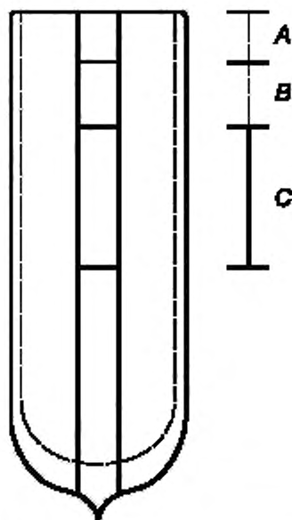
А — высота наполнения — 20 мм ниже верхней кромки; В — устанавливаемая 30-миллиметровая зона дефлакации; С — 50-миллиметровая зона измерения скорости дефлакации
