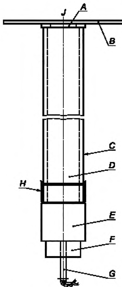
A — прокладки; B — контрольная пластина, C — стальная трубка; D — испытуемая химическая продукция; E — бустер, состоящий из циклотриметилентринитрамина/парафина или ТЭН/третилла; F — держатель детонатора; G — детонатор, H — пластмассовая мембрана, J — датчик скорости
