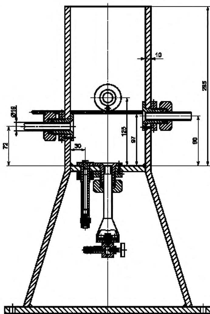
Рисунок 10 — Защитно-нагревательное устройство
