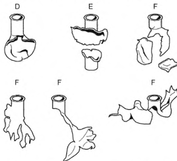
Рисунок 11 — Примеры разрушений видов «D», «E» и «F»
