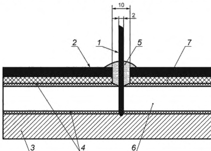
1 — термопара; 2 — наружная оболочка кабеля; 3 — токопроводящая жила; 4 — электропроводящие экраны; 5 — эластичный теплоизолирующий композит; 6 — изоляция; 7 — металлическая оболочка
