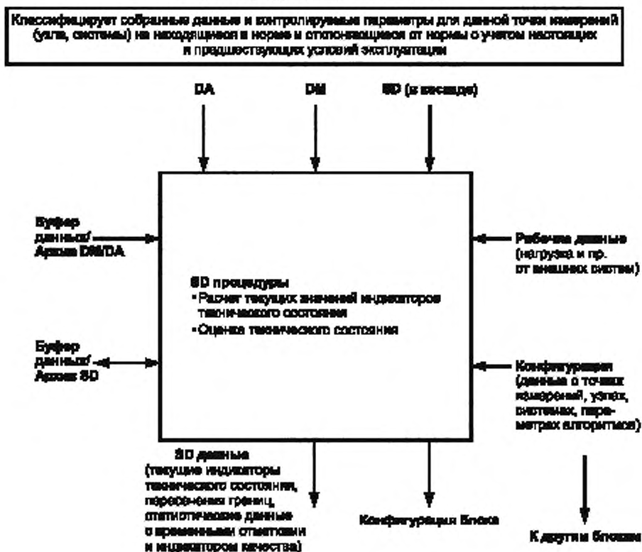
Рисунок 5 — Блок определения состояния
