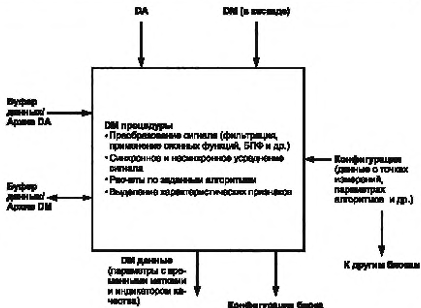
Рисунок 4 — Блок преобразования данных
