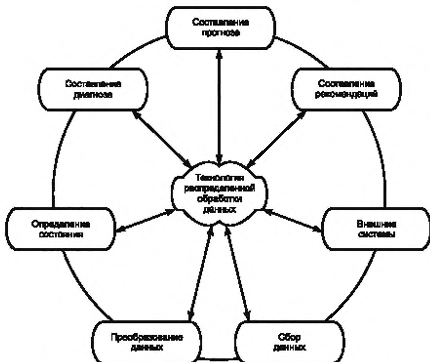
Рисунок 9 — Поток обработки данных в рамках стандартной архитектуры
