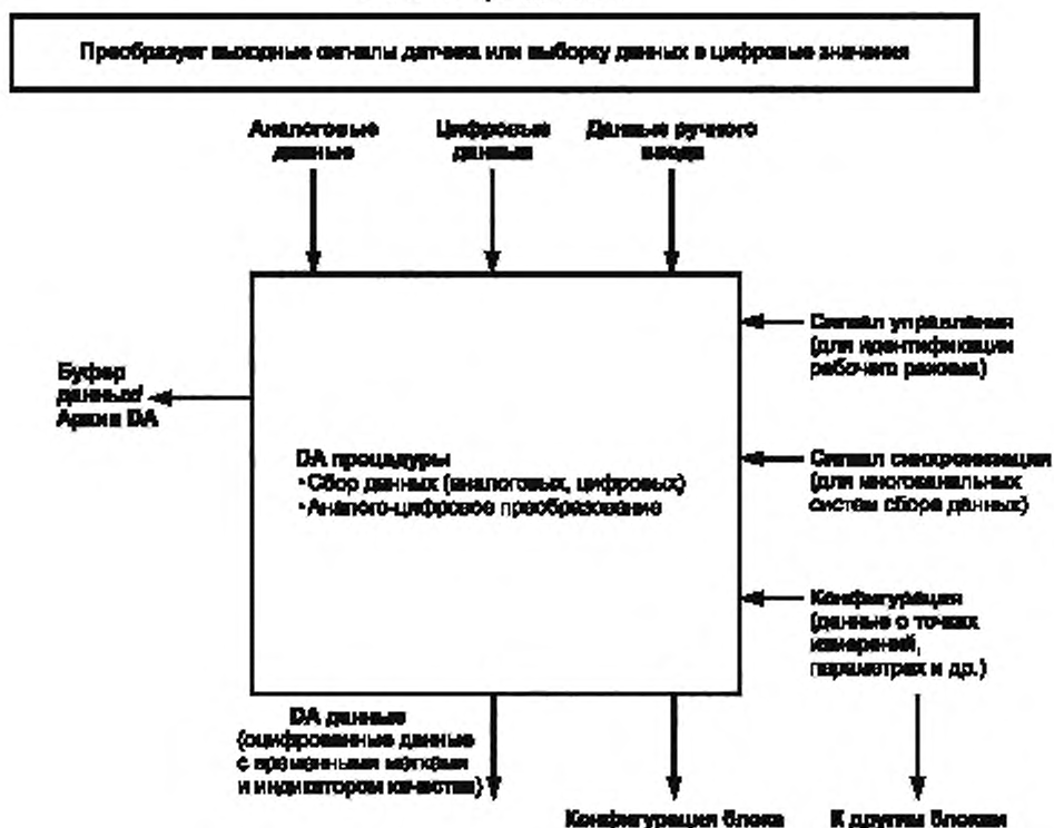
Рисунок 3 — Блок сбора данных
