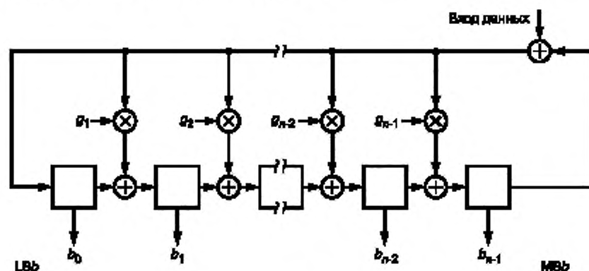
Рисунок А.1 — CRC генератор
