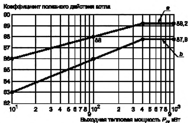
Рисунок 1 — Требования к коэффициенту полезного действия
