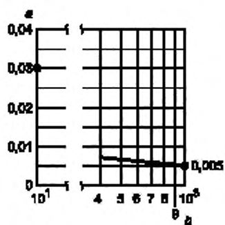
a — потери на холостом ходу; b — выходная тепловая мощность P_{\text{н}} , кВт Рисунок 5 — Потери на холостом ходу
