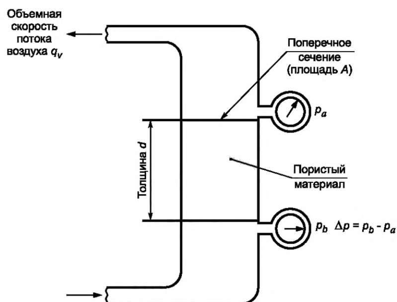
Рисунок 1 — Схема определения сопротивления продуванию постоянным потоком воздуха
