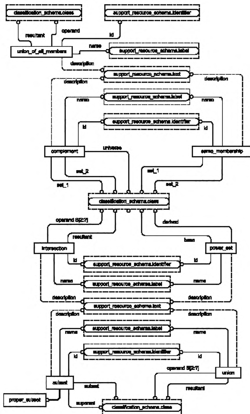
Рисунок D.2 — EXPRESS-G диаграмма схемы set_theory_schema
