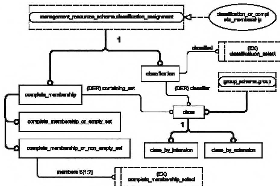
Рисунок D.1 — EXPRESS-G диаграмма схемы classification_schema
