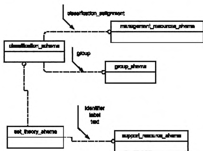
Рисунок 1 — Отношения между схемами по ИСО 10303-54
