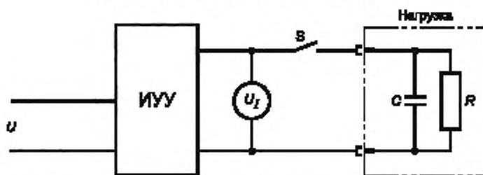
б) Схема для измерения тока с выключенной нагрузкой при установившемся режиме работы устройства управления
